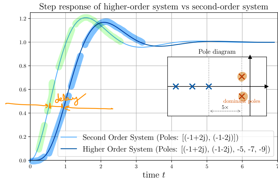
(b) complex conjugate poles
